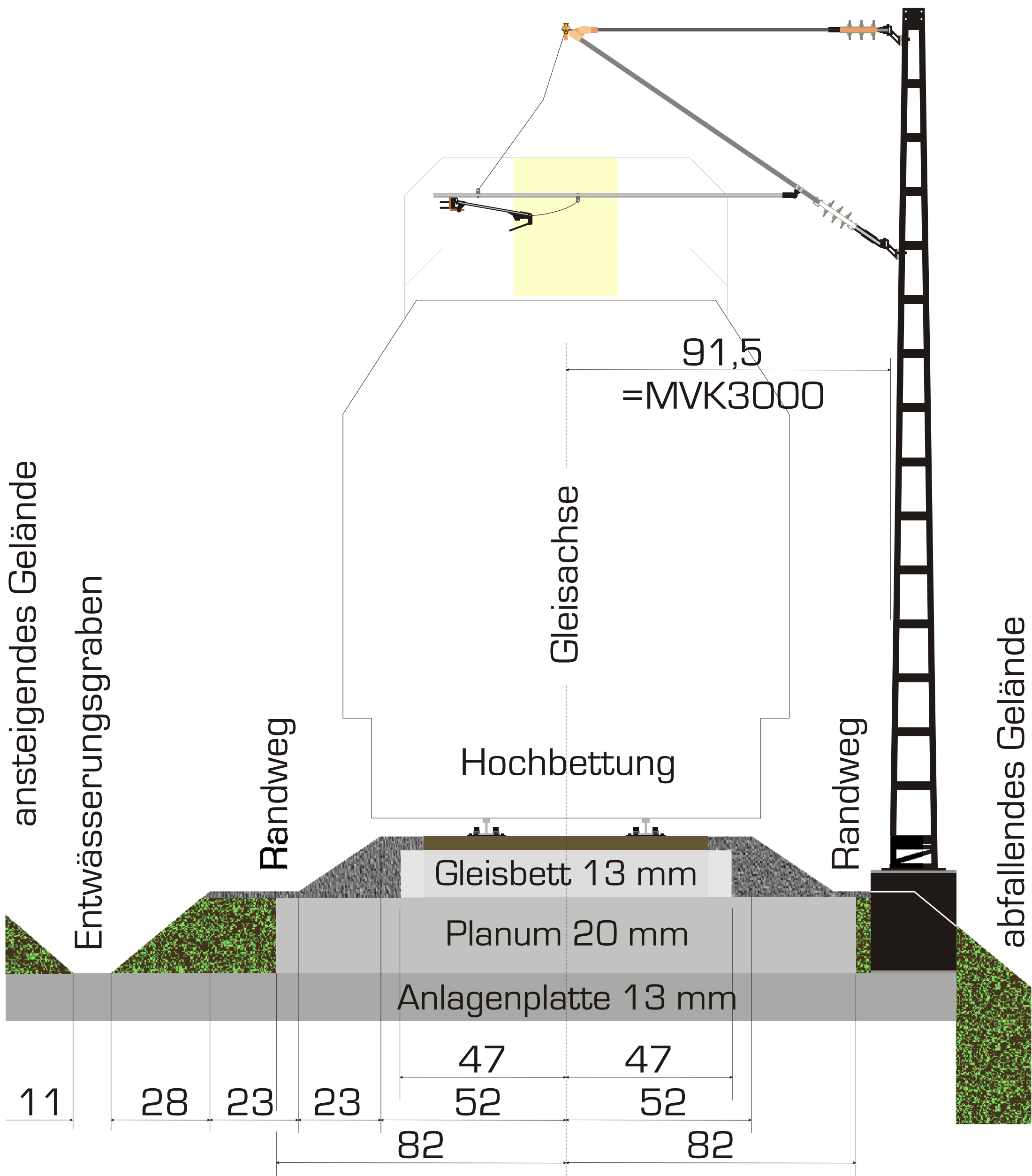
Vorbildgerechter eingleisiger Bahnkörper Deutsche Bundesbahn Maßstab 1:1 für Spur 1 Copyright © 2018 WENZ-MODELLBAU - Alle Rechte vorbehalten
